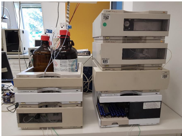
Slika 1: HPLC-FLD sistem med analizo vzorcev medu na sulfonamide
